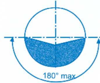
Askılı tip taşlama makinelerinde
