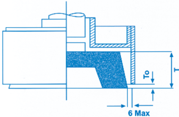
El taşlama aletlerinde çanak taşlar ile taşlama
