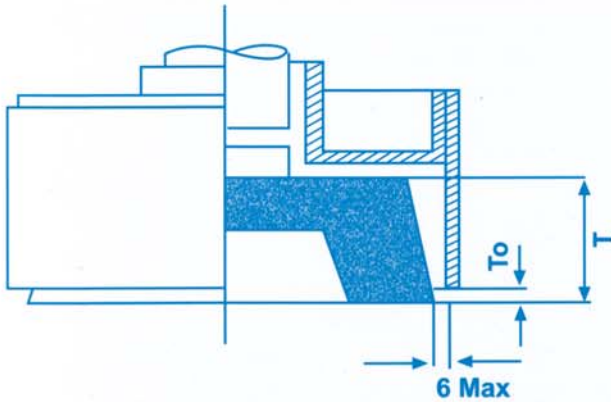
El taşlama aletlerinde çanak taşlar ile taşlama
