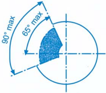
Duvar veya döşemeye tespit edilmiş taşlama makinelerinde
