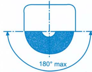
Yüksek basınçlı taşlama makinelerinde
