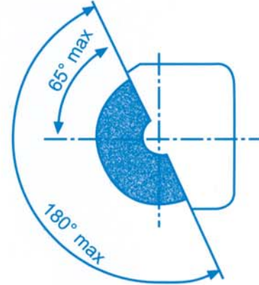
Silindirik taşlama makinaları
